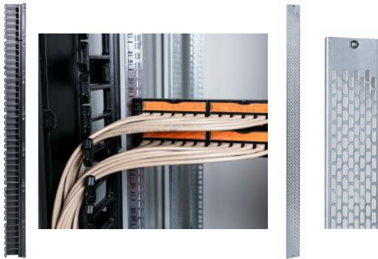
EVPM442 – izravno vođenje prespojnih kabela
